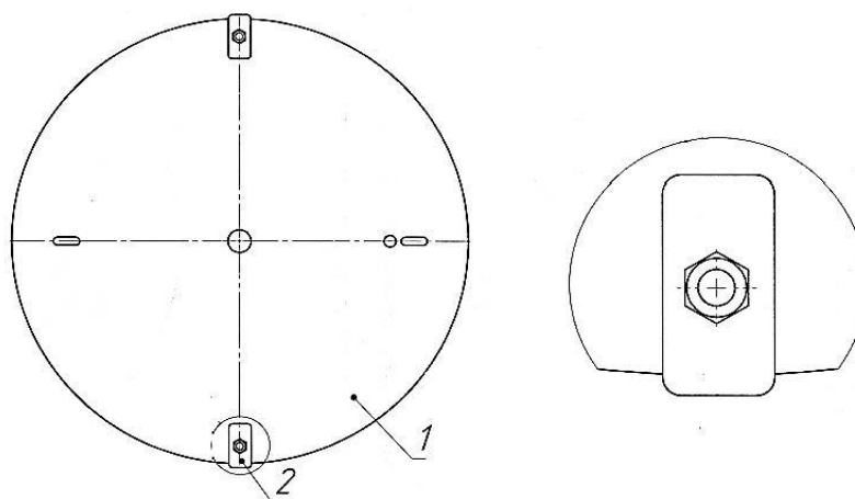
Рис. 3. Нижняя стальная крышка устройства УЗЛ-Л ССД с установленными заглушками. 1 – диск; 2 – задвижка с болтом и гайкой, вид сверху. Гайка запорного механизма на рисунке не показана.
